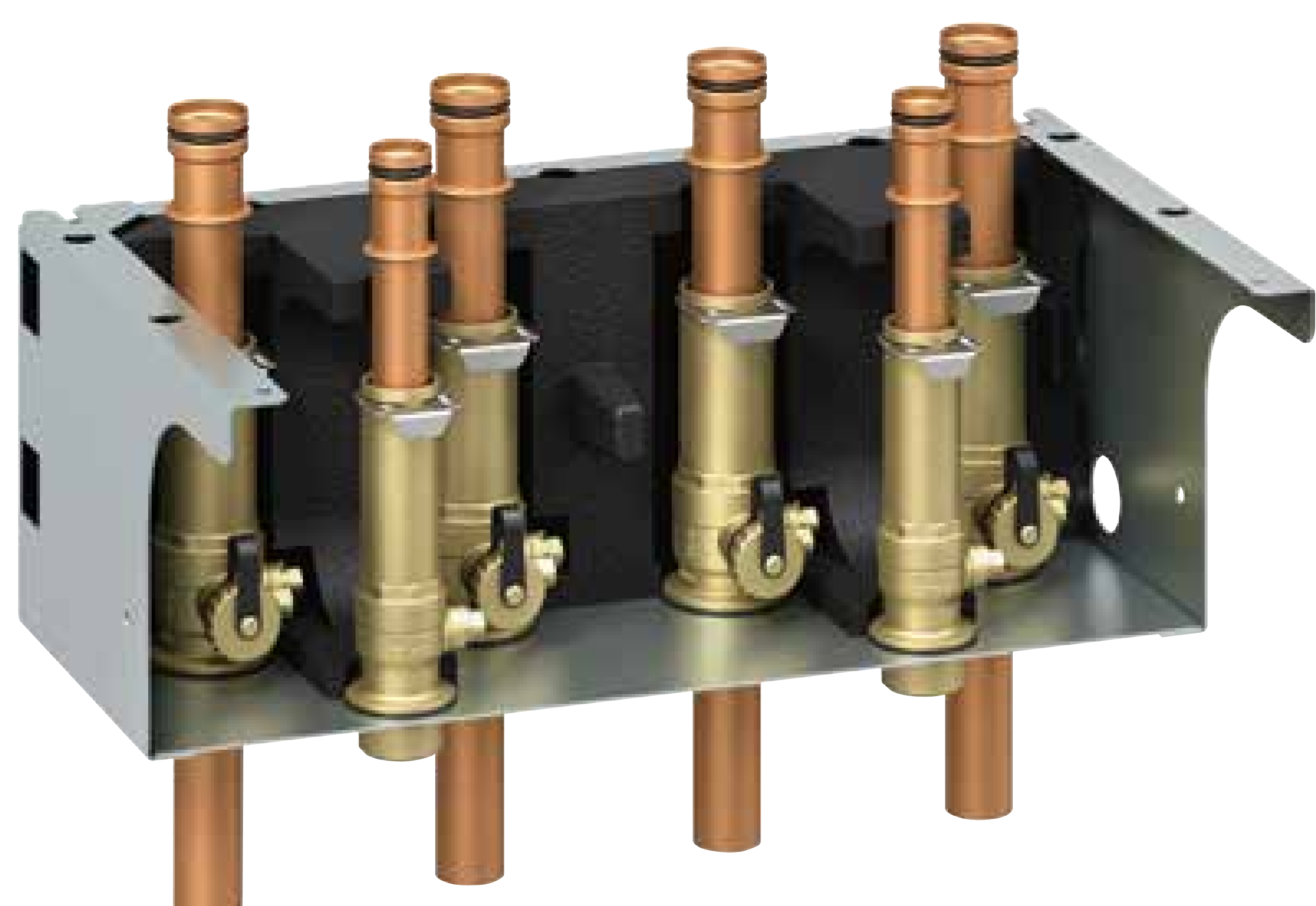
Montagehilfe Comfort mit G-Gewind 22/28 mm mit Zubehör
